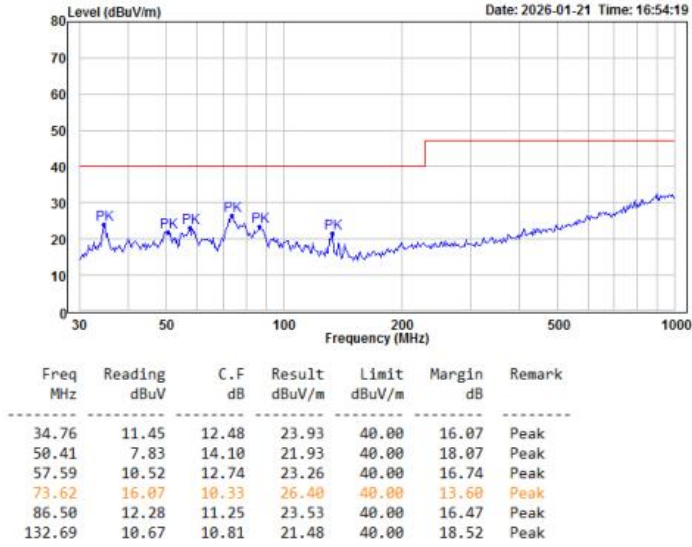
图 5-8 辐射测试垂直方向
