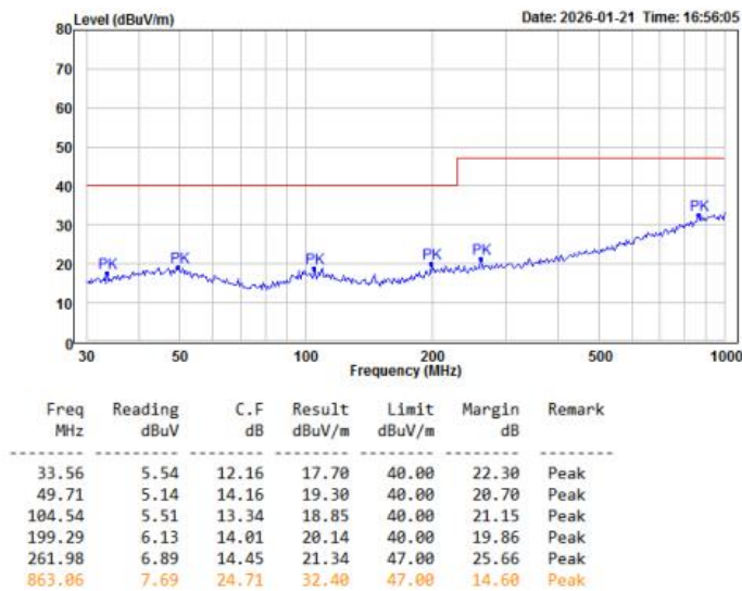
图 5-7 辐射测试水平方向
