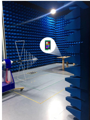
图 5-6 辐射测试图
